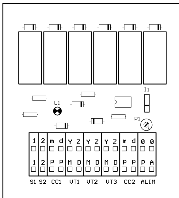
COMMANDES CENTRALISEES 2
